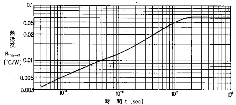
過渡熱抵抗(トランジスタ)特性
