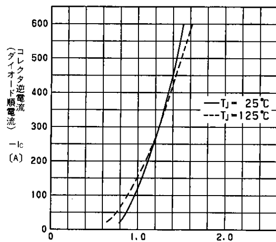
高速フリーホイーリングダイオード順電圧特性 Forward Voltage of Free Wheeling Diode
