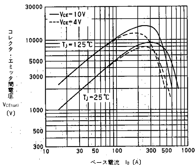
出力特性 Collector Output Characteristics
