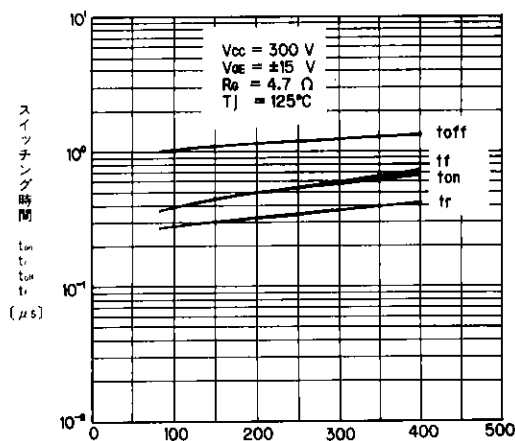
スイッチング時間—コレクタ電流特性 Switching Time vs. Collector Current
