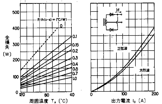
出力電流－全損失－周囲温度特性 Output Current - Total Loss - Ambient Temperature
