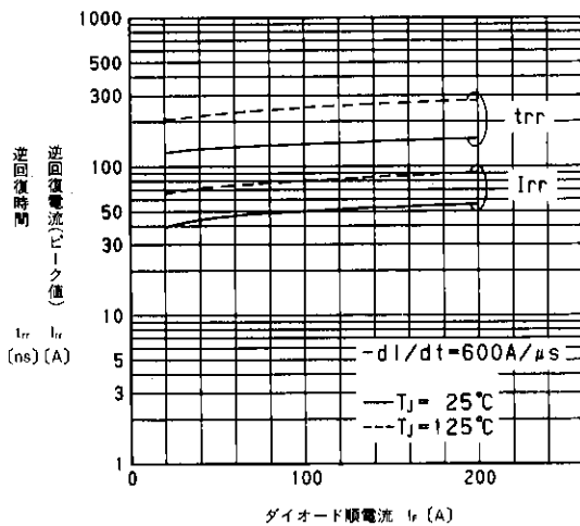
T_{rr} , I_{rr} - I_F 特性 T_{rr} , I_{rr} - I_F
