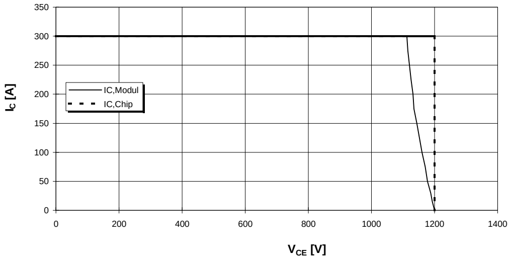
Sicherer Arbeitsbereich (RBSOA) Reverse bias safe operation area (RBSOA) V_{GE} = 15V, R_g = 5,6\text{ Ohm}, T_{vj} = 125^\circ C
