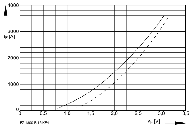
Bild / Fig. 6 Durchlaßkennlinie der Inversdiode (typisch) Forward characteristic of the inverse diode (typical) ..... t_{vj} = 25 \text{ °C} — t_{vj} = 125 \text{ °C}
