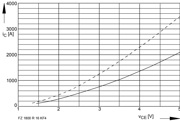
Bild / Fig. 1 Kollektor-Emitter-Spannung im Sättigungsbereich (typisch) Collector-emitter-voltage in saturation region (typical) V_{GE} = 15 \text{ V} ..... t_{vj} = 25 \text{ °C} — t_{vj} = 125 \text{ °C}
