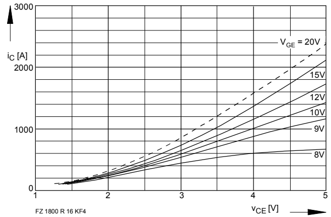
Bild / Fig. 2 Kollektor-Emitter-Spannung im Sättigungsbereich (typisch) Collector-emitter-voltage in saturation region (typical) t_{vj} = 125 \text{ °C}
