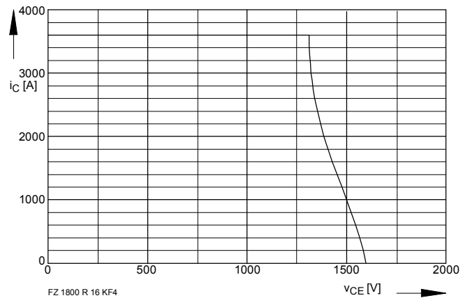
Bild / Fig. 4 Rückwärts-Arbeitsbereich Reverse biased safe operating area t_{vj} = 125 \text{ °C}, V_{LF} = V_{LR} = 15 \text{ V}, R_G = 1.2 \Omega
