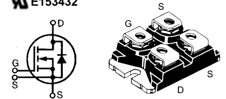
miniBLOC, SOT-227 B (IXFN)
