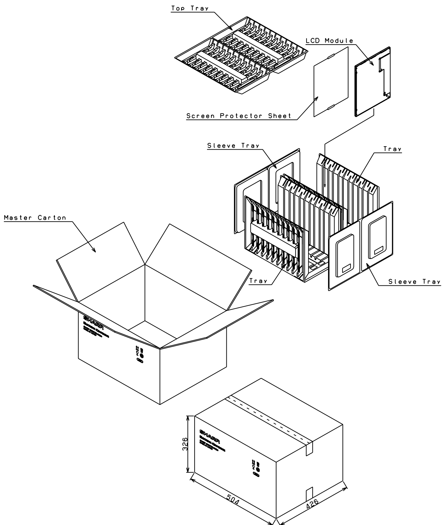
图3. 包装形态图
