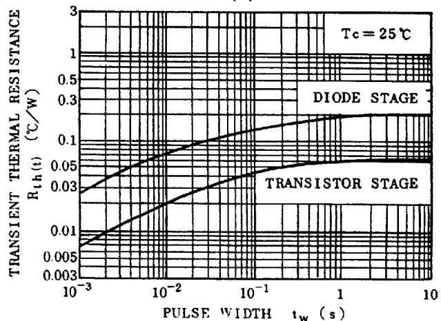
R_{th}(t) - t_w
