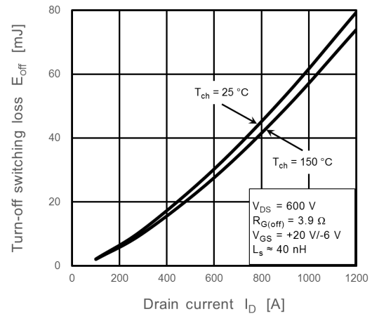
Fig. 8.8 E_{off} - I_D
