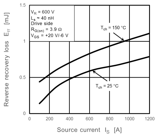
Fig. 8.9 E_{rr} - I_S
