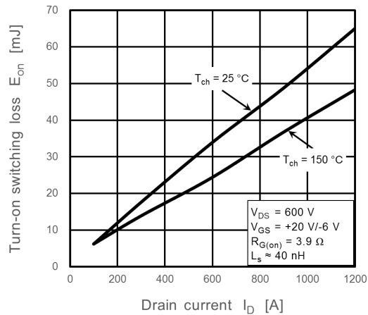
Fig. 8.7 E_{on} - I_D
