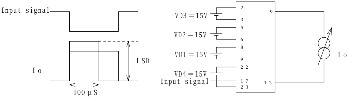
Fig 5 : I SD
